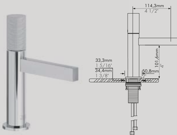
FV181/J2K Juego monocomando para lavatorio con desagüe "soft touch". PC-BB-BG-BK-BN PB-BHB-UPB-PN-SGR
