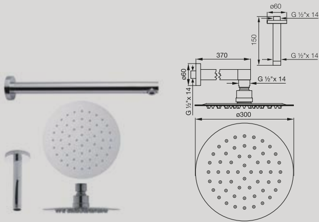
FR126.04.1.0 Ducha redonda de 300 mm. con brazos de pared y de techo. BB-BG-PB-CR BK-SGR-BN-UPB BHB-PN
