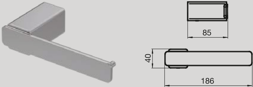
FV167/J5 Portarrollo. PC-FB
