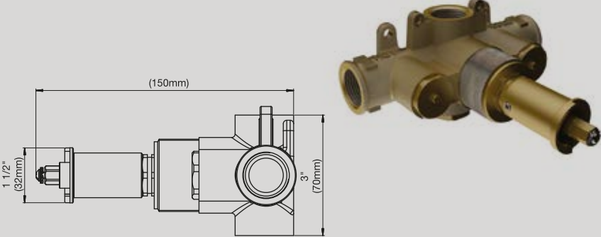
FV217.BASE Base para unidad termostatica de gas 3/4". Latón
