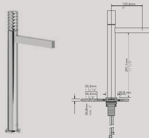
FV181.02/J2D Juego monocomando para lavatorio, para bachas tipo Vessel, con desagüe soft touch. PC-BB-BG-BK-BN PB-BHB-UPB-PN-SGR
