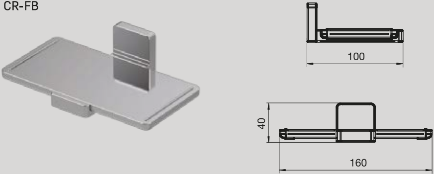
FR168/J5 Jabonera. CR-FB
