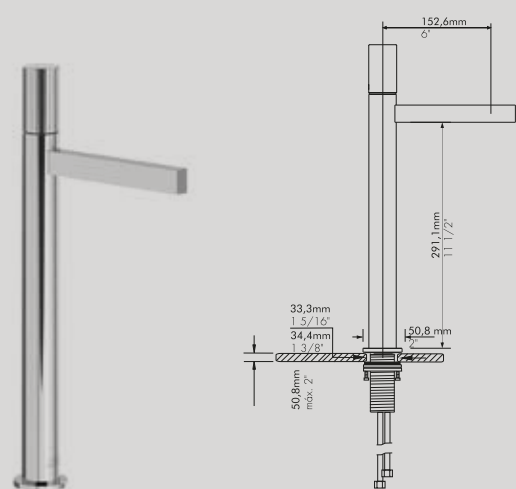
FV181.02/J2V Juego monocomando para lavatorio, para bachas tipo Vessel, con desagüe soft touch. PC-BB-BG-BK-BN PB-BHB-UPB-PN-SGR
