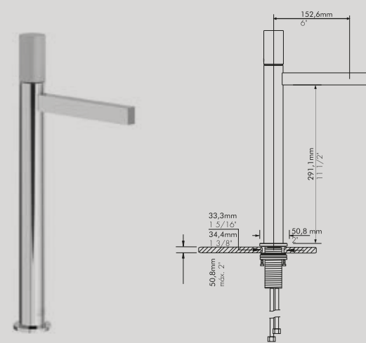
FV181.02/J2K Juego monocomando para lavatorio, para bachas tipo Vessel, con desagüe soft touch. PC-BB-BG-BK-BN PB-BHB-UPB-PN-SGR
