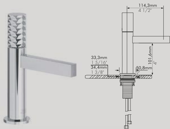
FV181/J2D Juego monocomando para lavatorio con desagüe "soft touch". PC-BB-BG-BK-BN PB-BHB-UPB-PN-SGR
