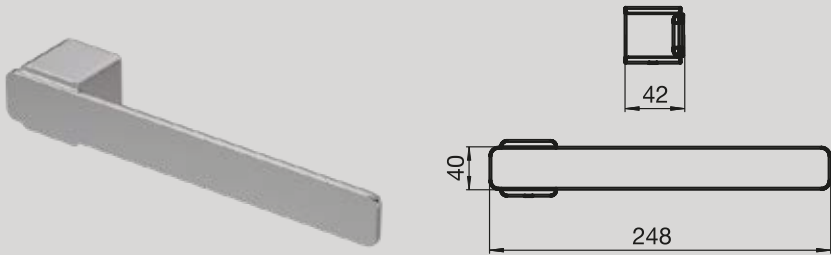
FV163/J5 Toallero corto. PC-FB
