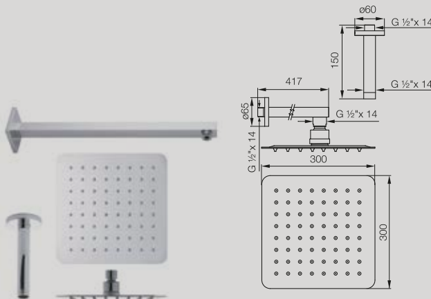
FR126.05.1.0 Ducha cuadrada de 300 mm. con brazos de pared y de techo. BB-BG-PB-CR BK-SGR-BN-UPB BHB-PN
