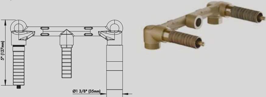
FI203.BASE Base para juego de lavatorio de pared. de gas 1/2". Latón
