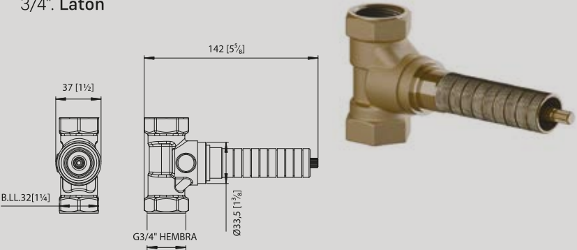
FI480.BASE-19 Base de llave de paso armada completa de gas 3/4". Latón
