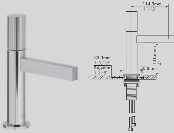
FV181/J2V Juego monocomando para lavatorio con desagüe "soft touch". PC-BB-BG-BK-BN PB-BHB-UPB-PN-SGR
